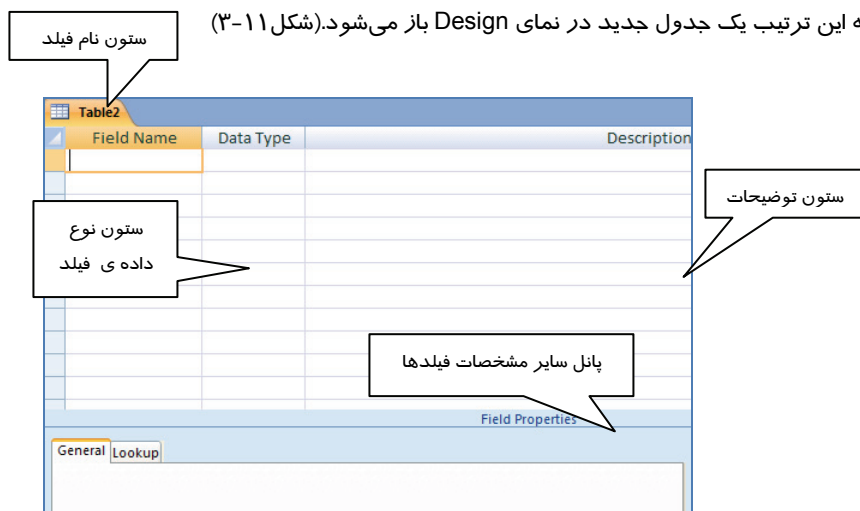
(شکل ۱۱-۳ نمای Design جدول جدید)
