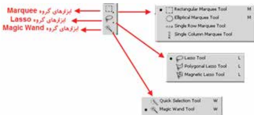
شکل ۱-۱۷ ابزارهای انتخاب
