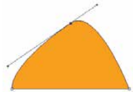
شکل ۷-۲۲- نقاط Smooth
