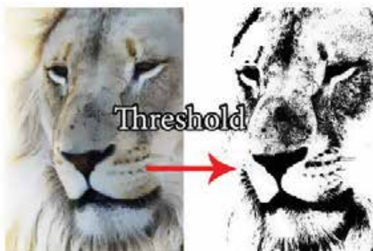
شکل ۲۴-۲۵ دستور Threshold
