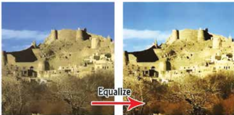
شکل ۲۴-۲۴ دستور Equalize
