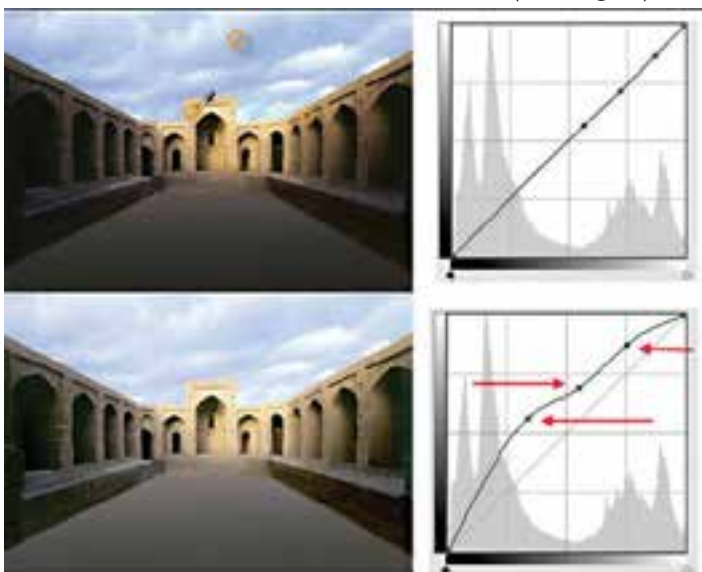
شکل ۱۲-۲۴ منحنی Curve
