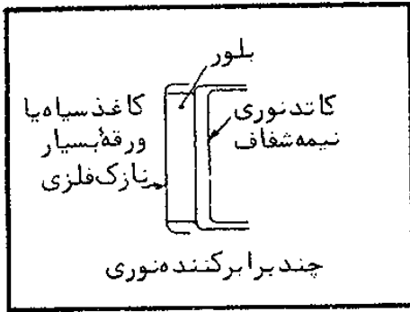
شکل ۳۲- پارتیکول های هسته ای از کاغذ سیاه یا صفحه فلزی (که برای جلوگیری از عبور نور است) می گذرند و در بلور نفوذ می کنند. این بلور برای هر پارتیکول برقی می فرستد که به وسیله چند برابر کننده نوری که بلور روی آن چسبیده است، آشکار می شود.
