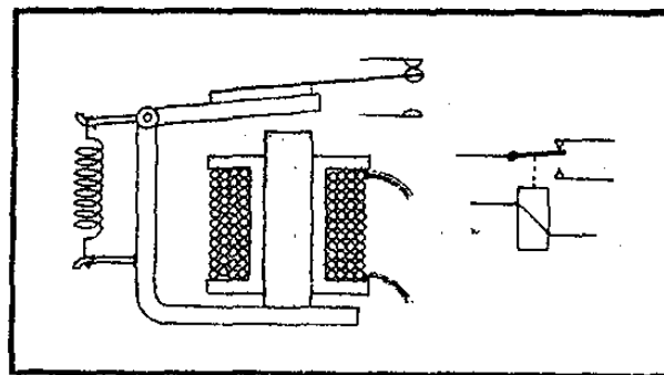
شکل ۹۲ - يك رله (که به صورت اختصاری در سمت چپ نشان داده شده). شامل يك قرقره است که يك میدان مغناطیسی ایجاد می کند و تیغه را جذب کرده و باعث می شود که يك انصالی، که اتصال کار نام دارد، باز یا بسته شود.
