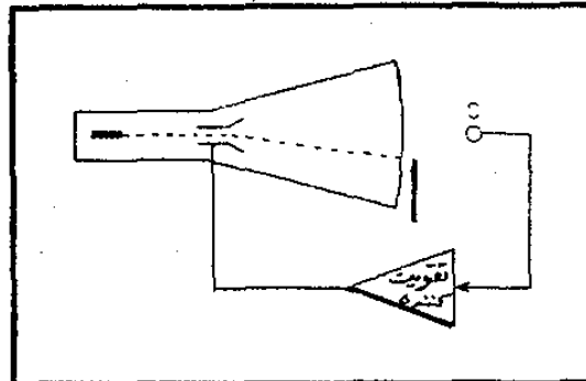
شکل ۱۴۳- يك مثال برای سیستم تابع: سلول فتوالکتریک C بر حسب آنکه مقوا چگونگی بین سلول و اسپات قرار گرفته باشد، کم و بیش نور اسپات لامپ کاتدی را جذب می کند، این سلول تغییر وضعیت اسپات را فرمان می دهد.
