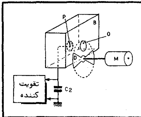
شکل ۱۰ - صفحه گرد P، که درجه سربسته B قرار دارد، در برابر یک سوراخ O قرار گرفته است که صفحه گردان D آنرا سد و باز می‌کند و به این ترتیب اثر میدان الکتريکی P به همان آهنک مدولاسیون پیدا می‌کند.
