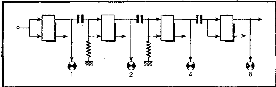
شکل ۱۱۵ - به وسیله يك سلسله قپان که هر کدام دیگری را فرمان می‌دهد، يك شمارگر دو تایی درست می‌کنند، درحالی‌که وضع هر قپان به وسیله يك لامپ مشخص می‌شود.
