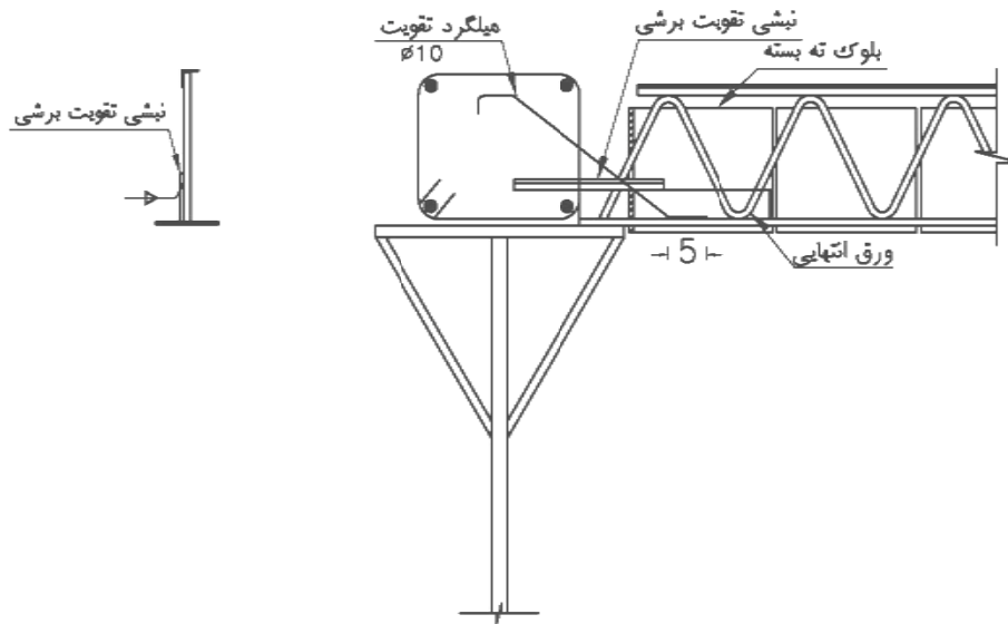
شکل ۳-۱۳- نحوه تعبیه نشی در محل اتصال (تقویت برشی)
