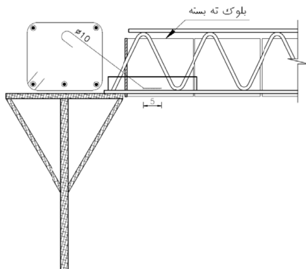
شکل ۳-۱۱- نحوه‌ی کارگذاری قالب چوبی در محل اتصال تیرچه به تیر فولادی (حالت اول)
