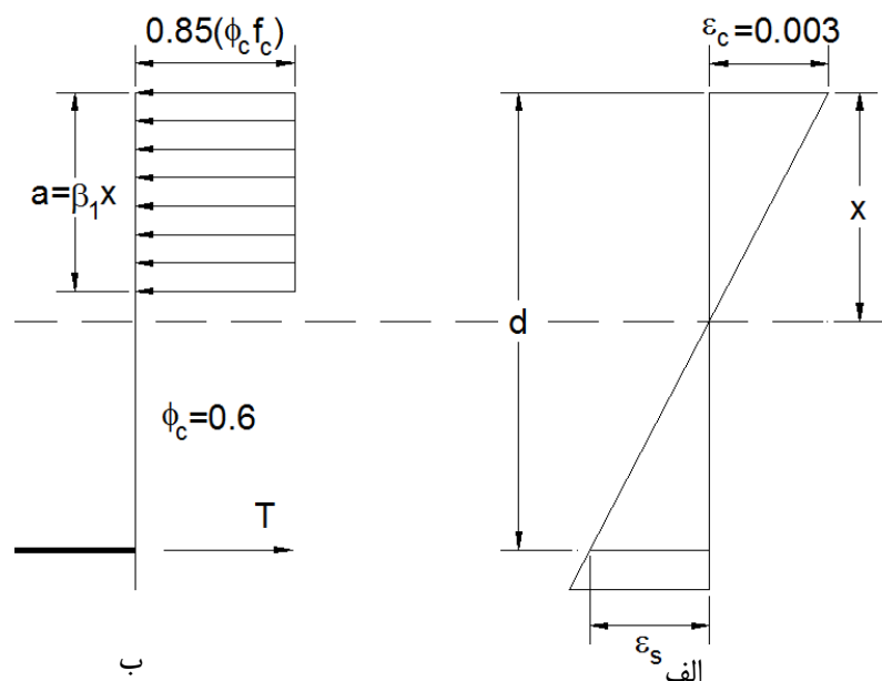
شکل پ ۲-۳- بلوک تنش مستطیلی
