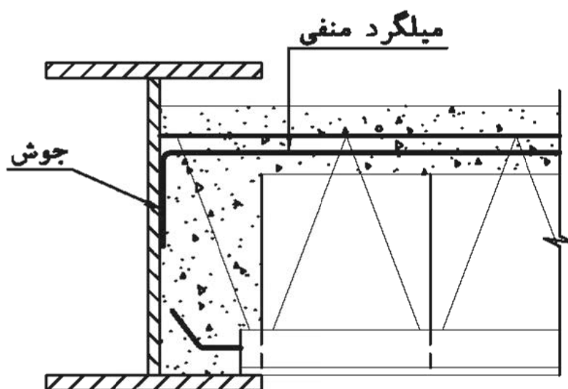
شکل ۵-۱۶- استقرار سقف تیرچه و بلوک روی تیر باربر فولادی با ارتفاع بیشتر از ضخامت سقف، در تکیه‌گاه کناری
