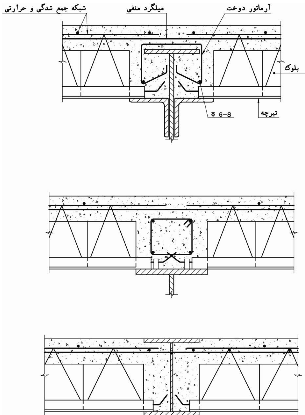
شکل ۵-۱۱- استقرار سقف تیرچه و بلوک روی تیرآهن، با ارتفاع مساوی و یا با ارتفاع کمتر از ضخامت سقف تیرچه و بلوک
