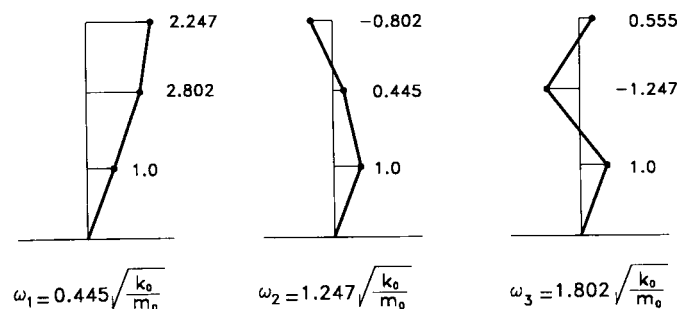
شکل ۱. ۲۴ فرکانس و اشکال مدی یک سازه سه درجه
